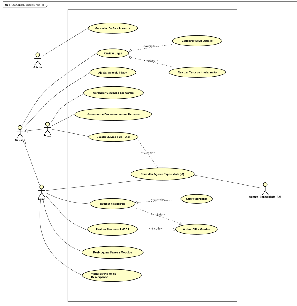
Figura 13 – Diagrama de Casos de Uso: Visão Geral
